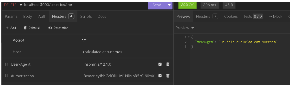
Tela #5: Exemplo de Rota com geração de Log:
